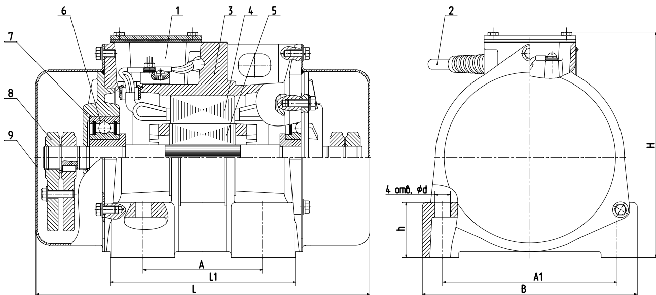
Рисунок 2. Вибратор ИВ–05-16.
