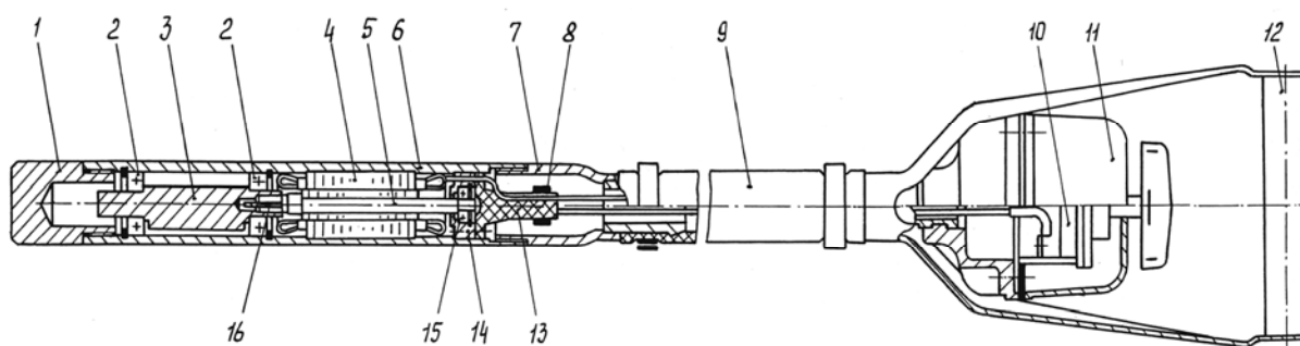
Рисунок 3. Вибратор ИВ – 78.
