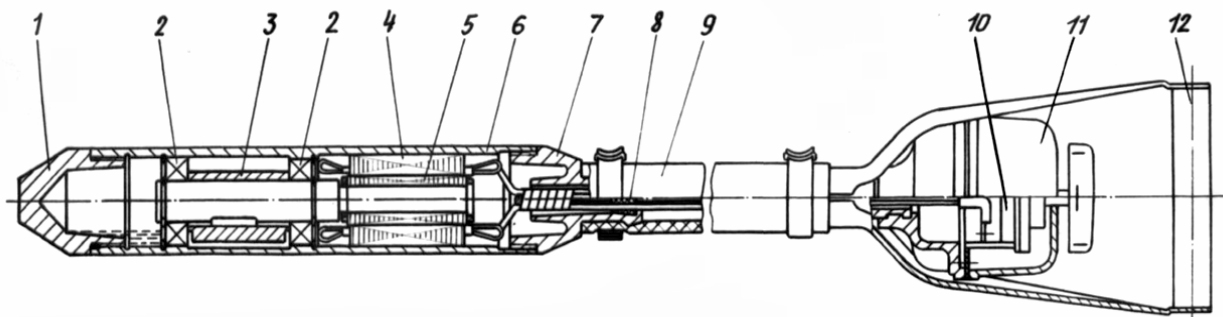
Рисунок 4. Вибратор ИВ – 102А.
