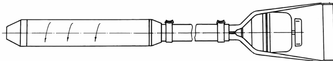
Рисунок 6. Схема установления направления вращения вала ротора вибраторов ИВ-78, ИВ-102А.
